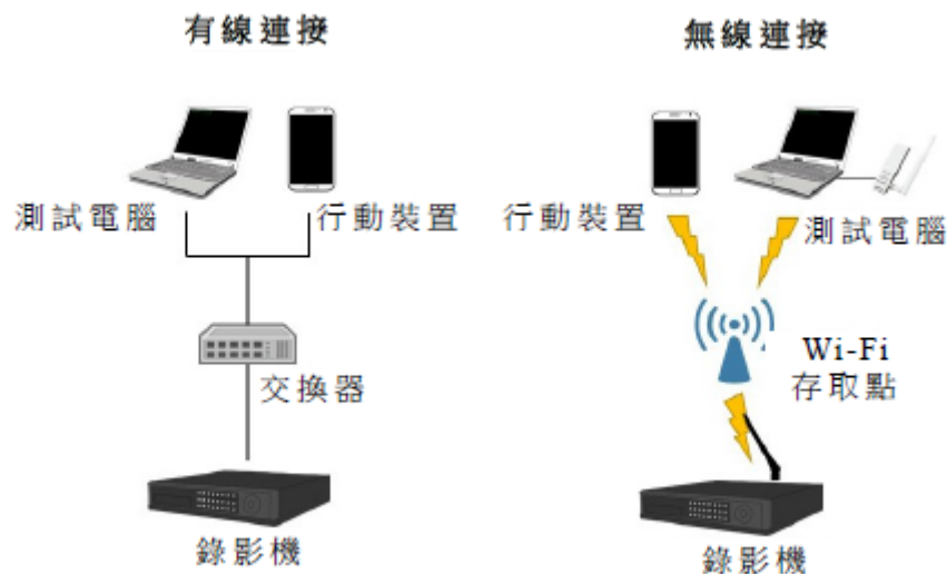
圖2 測試布局示意圖
